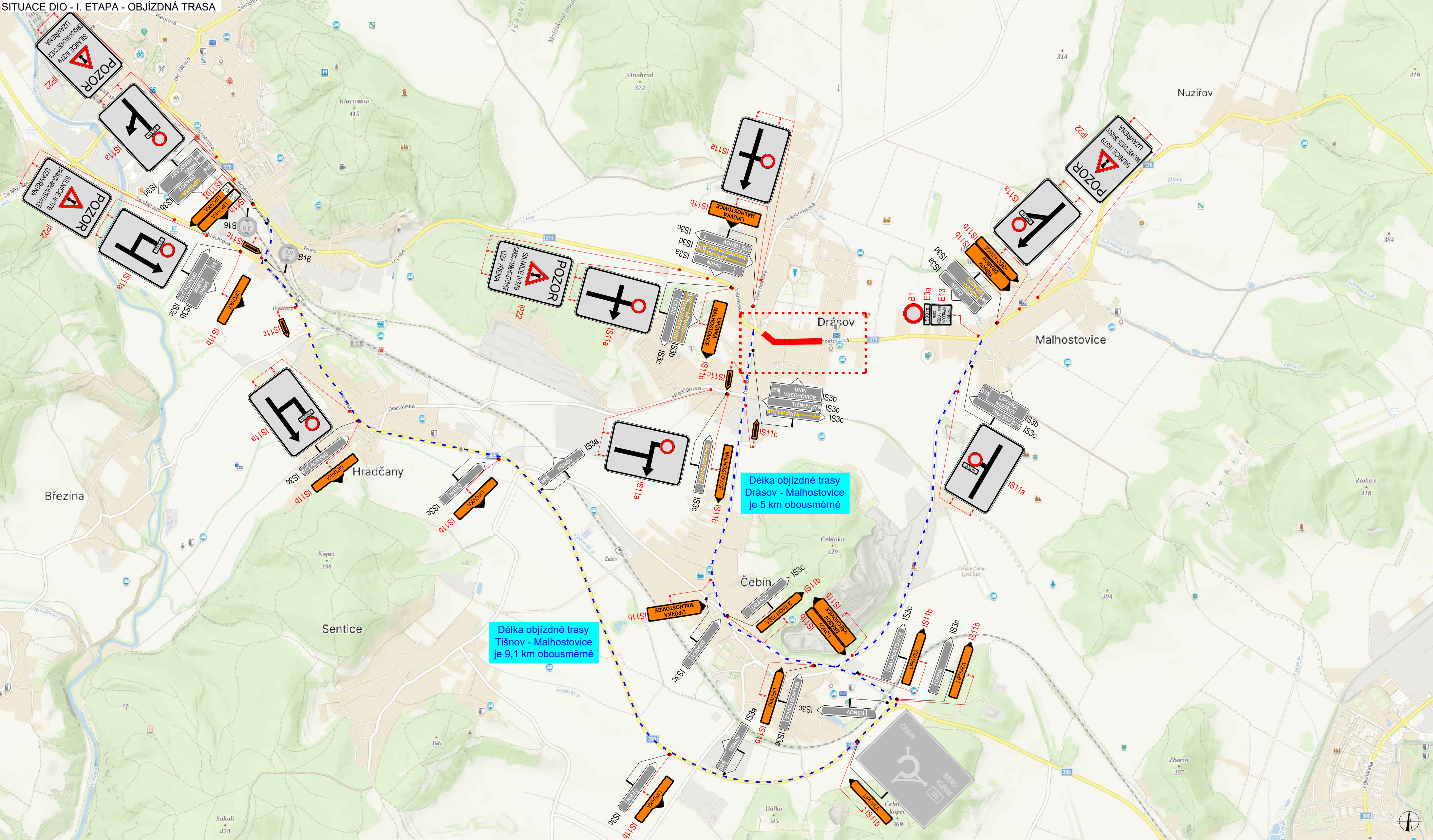
SITUACE DIO - I. ETAPA - DETAIL UZAVÍRKY
